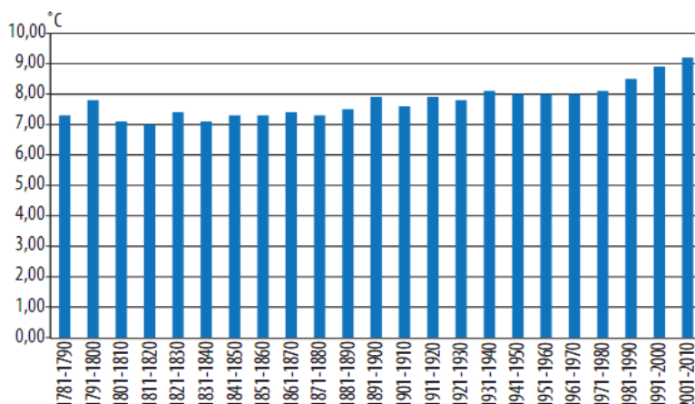
Ryc. 1. Wartości średniej rocznej temperatury powietrza w dziesięcioleciu na podstawie pomiarów stacji meteorologicznej Warszawa – Obserwatorium w latach 1781–2010 [źródło: Stan środowiska w Polsce – Raport 2014, GIOŚ 2014 za IMGW- PIB].
