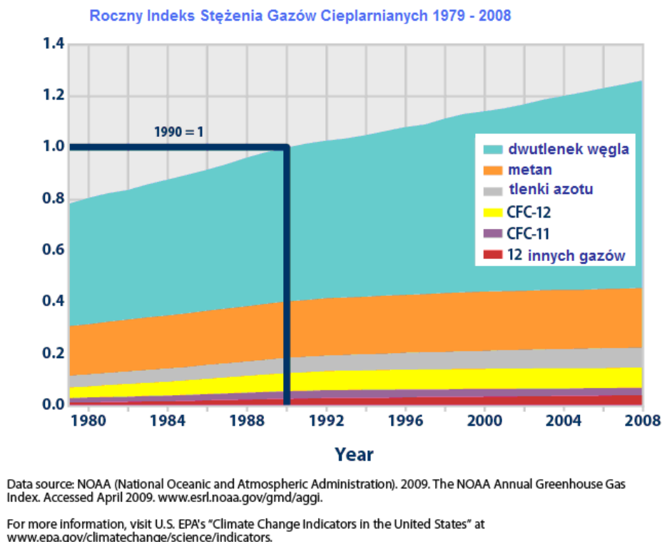
Ryc. 3. Przyrost ilości gazów cieplarnianych w atmosferze w latach 1979–2008. [źródło: NOAA – Narodowa Administracja Oceanów i Atmosfery USA]
