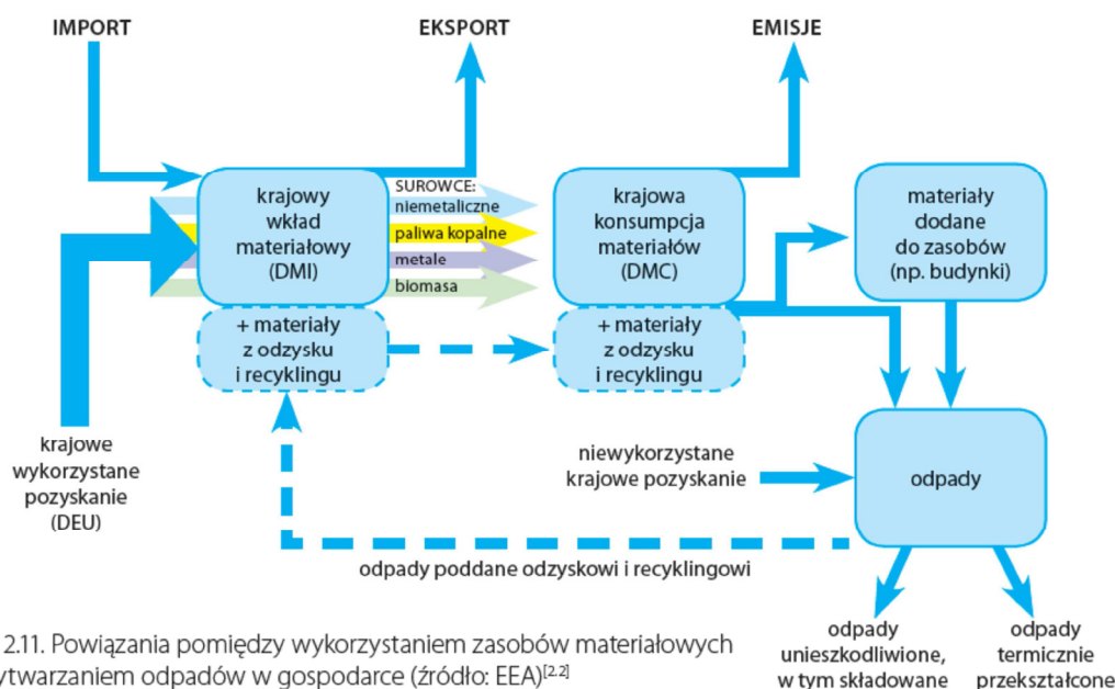
Ryc. 6. Powiązania pomiędzy wykorzystaniem zasobów materiałowych a wytwarzaniem odpadów w gospodarce. Źródło: GIOŚ, Stan środowiska w Polsce, Raport 2014, za EEA 2013 Environmental indicator Report 2012
